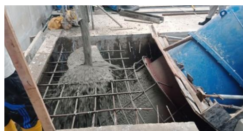
川への放流パイプの固定工事
